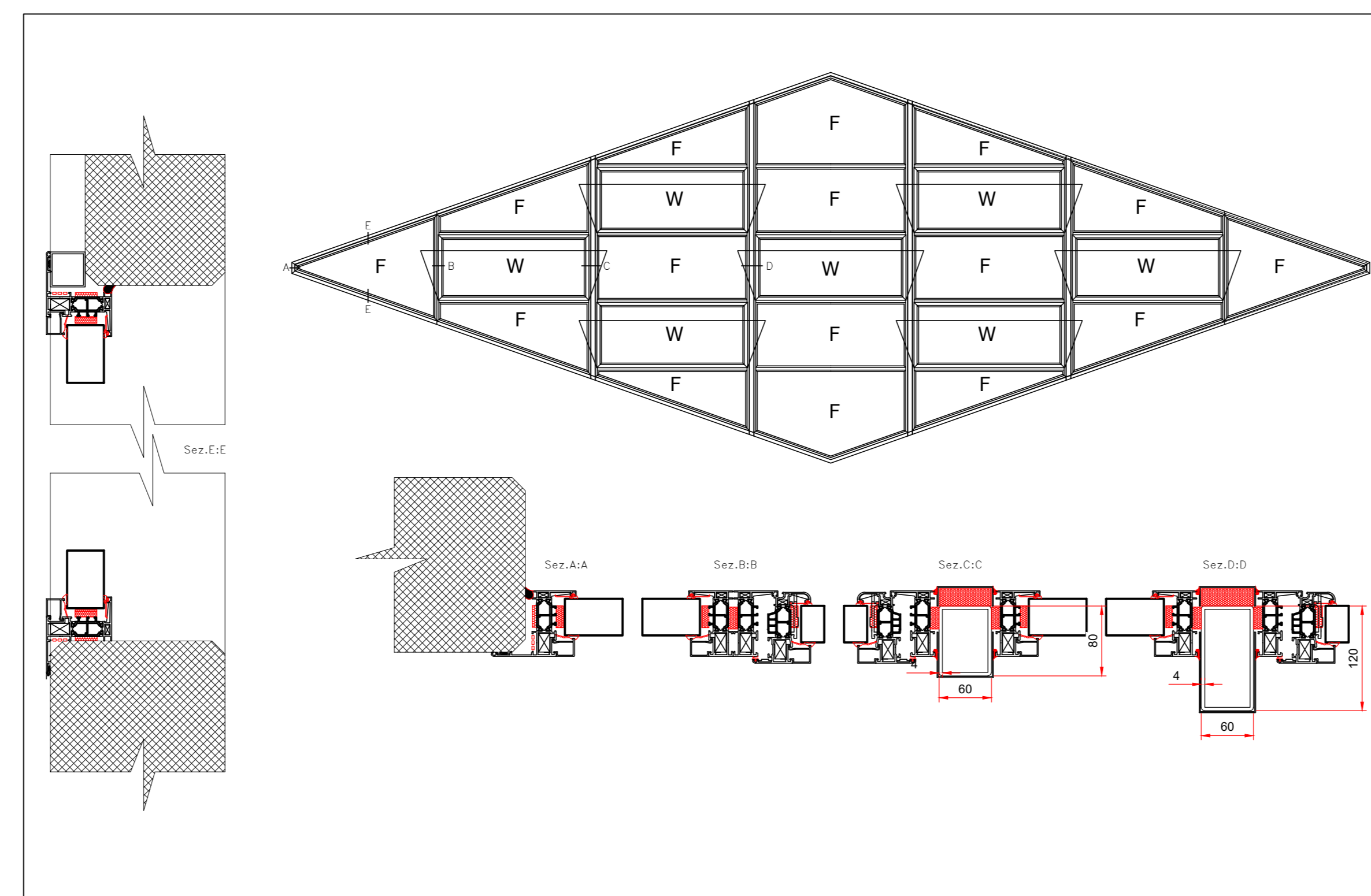
SEZIONI TIPO 1:5
