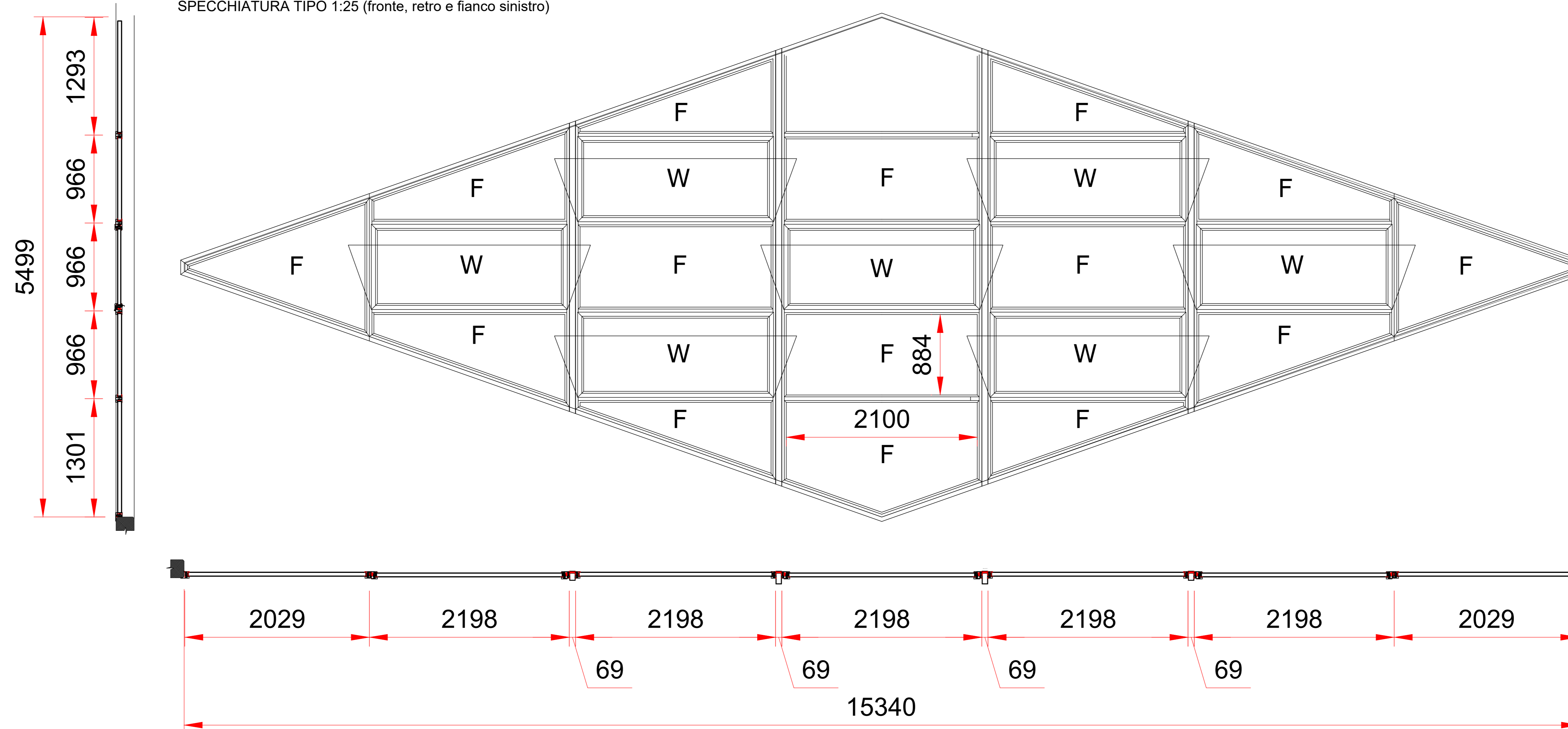
SPECCHIATURA TIPO 1:25 (fronte, retro e fianco sinistro)
