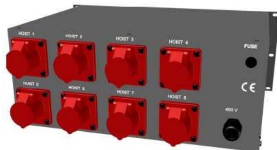
Vista del retro del controllore
