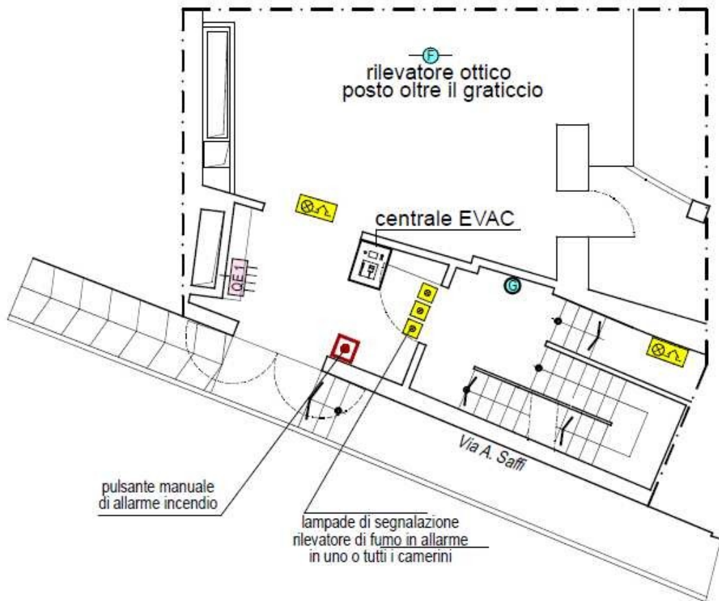
Indicazione planimetrica presenza altri impianti zona palcoscenico
