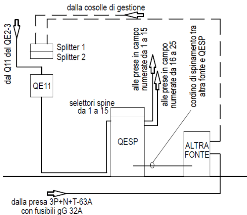
Schema a blocchi per il collegamento con il quadro di spinamento (QESP)
