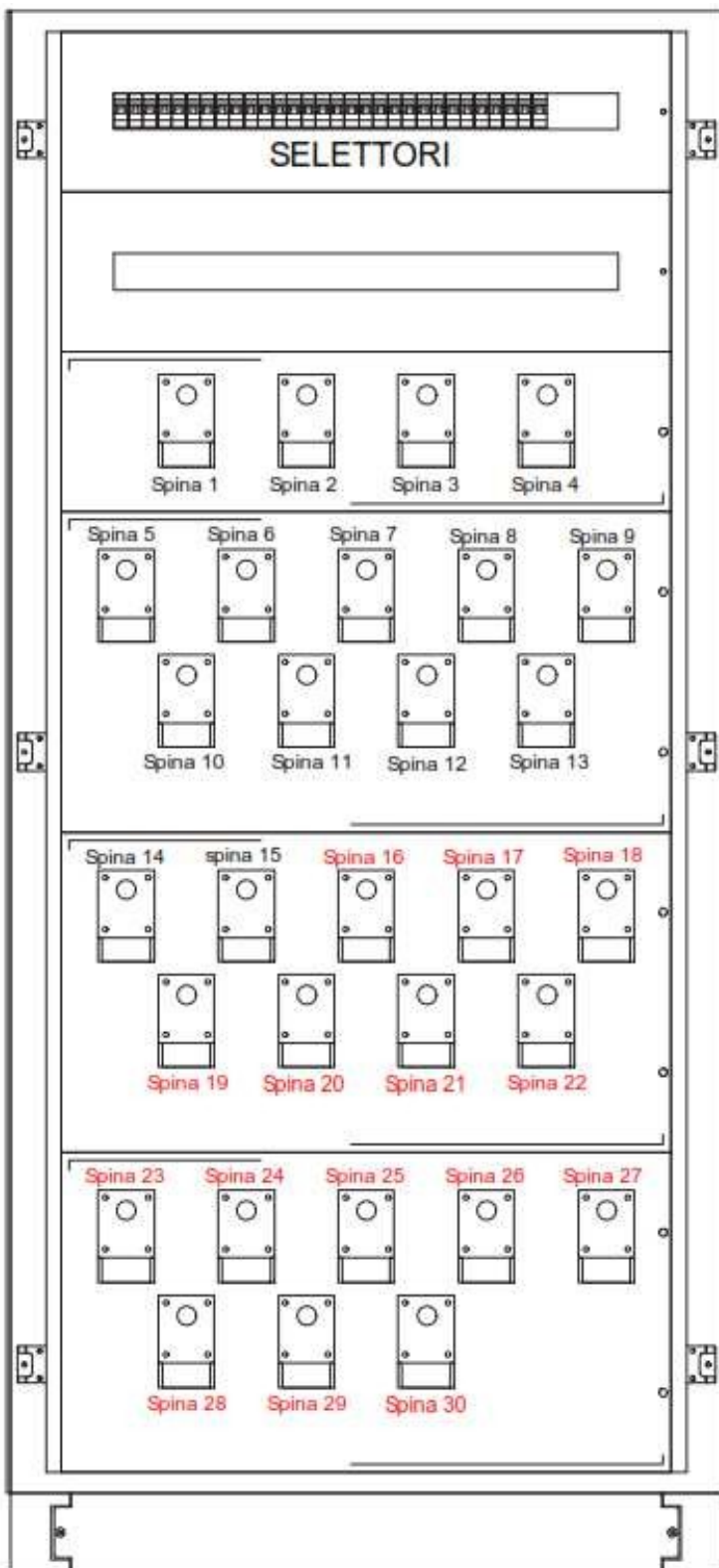
Fronte quadro di spinamento
